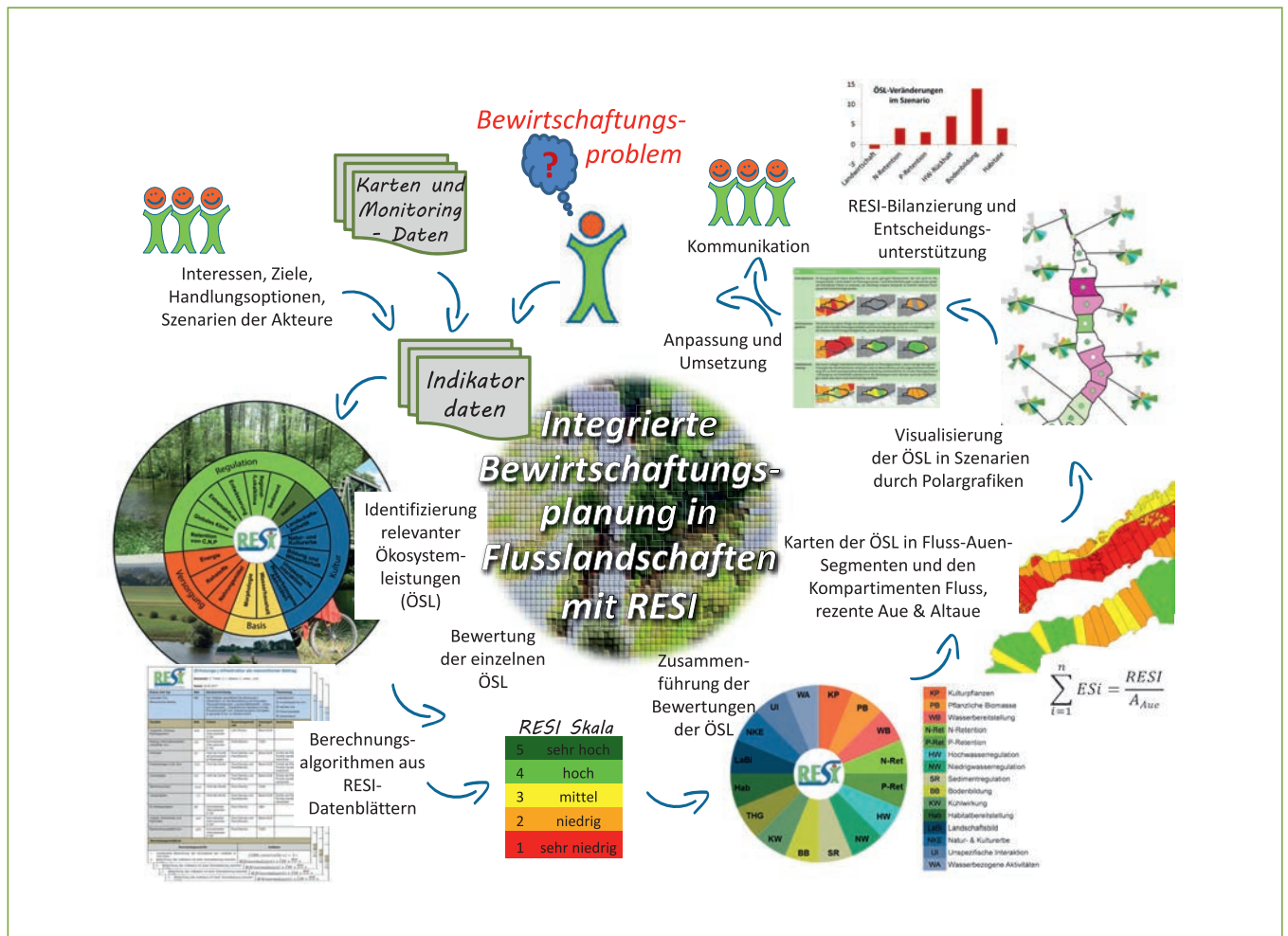
Abb. 2: Übersicht über das RESI-Verfahren zur Bewertung von Ökosystemleistungen (ÖSL) von Flusslandschaften. (Grafik: RESI-Projekt, Auenabgrenzung: Bundesamt für Naturschutz 2009, ©GeoBasis-DE/BKG 2016)
