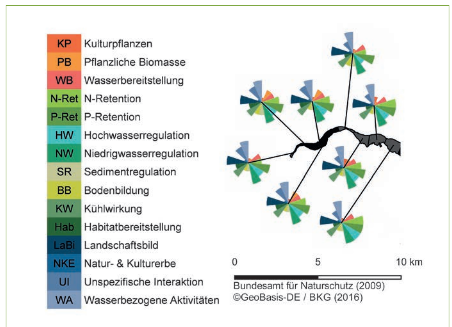
Abb. 3: Visualisierung der fünfstufigen Bewertungen der Verfügbarkeit der einzelnen Ökosystemleistungen in jedem Fluss-Auen-Segment durch zugeordnete Polardiagramme. (Grafik: RESI-Projekt)
