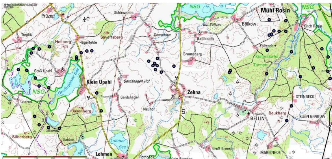
Abb. 2: Das Untersuchungsgebiet mit den untersuchten Probekreisen südlich von Güstrow. (Nicht dargestellt ist ein weiterer PK nördlich von Güstrow).
