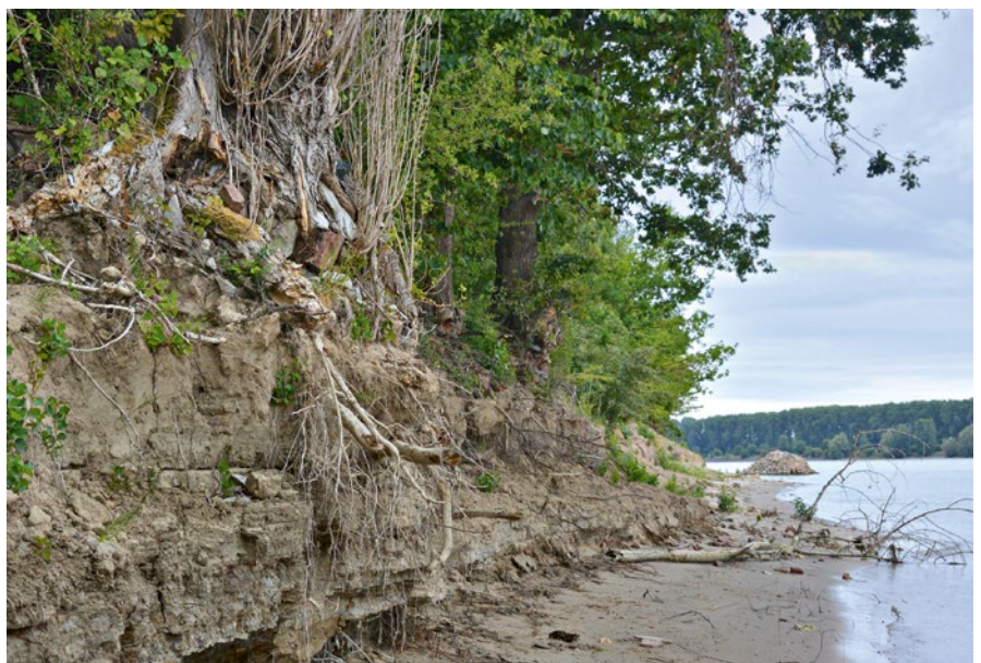
Abb. 1, oben, links: Rückbau eines versteinerten Rheinufer durch Entnahme der Wasserbausteine. (Foto: WSA Oberrhein, Mannheim, 2019)
