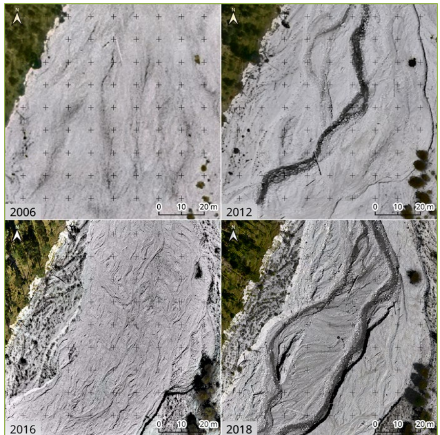
Abb. 4: Anhand von Luftbildern der Jahre 2006, 2012, 2016 und 2018 wird die Wechselfolge von Abtragung und Auflandung im Kernuntersuchungsgebiet deutlich. (© Bayerische Vermessungsverwaltung)
