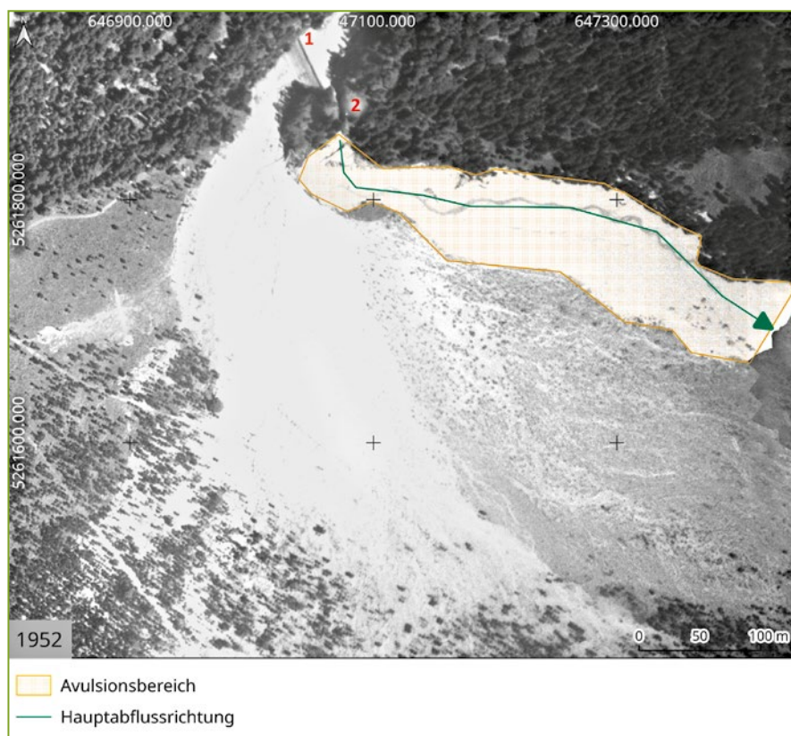
Abb. 2: Auf dem Luftbild von 1952 sind die Franzosenmauer (1) und der Durchstich (2) sowie die nach Südosten entwässernde Friederlaine zu erkennen. (© Bayerische Vermessungsverwaltung)
