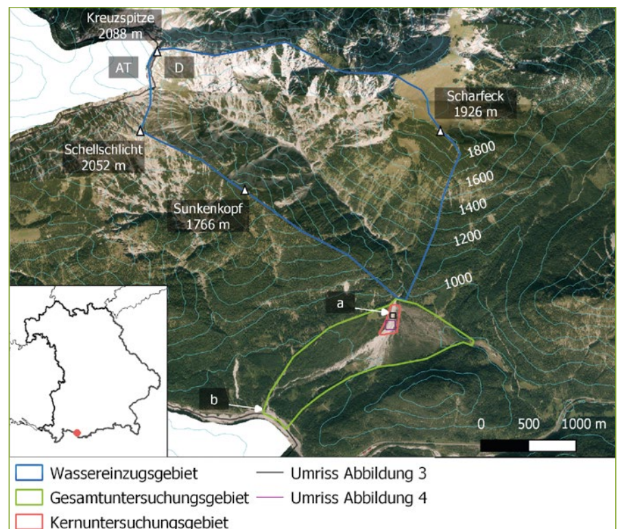
Abb. 1: Lage des Gesamt- und Kernuntersuchungsgebietes, des Wassereinzugsgebietes, der Umriss der Beispielflächen aus Abbildung 3 und Abbildung 4 sowie der bestehenden Uferverbauung (a) und der Kiesentnahme (b). Höhenlinien basierend auf SRTM-Daten; digitales Orthophoto (DOP80): © Bayerische Vermessungsverwaltung.
