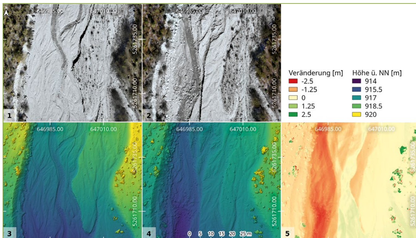
Abb. 3: Der Vergleich der Drohnenaufnahmen von 2016 und 2019 (1 und 2) sowie der errechneten Geländemodelle (3 und 4) und der daraus abgeleiteten morphologischen Veränderungen (5) belegt die Eintiefungstendenz im Kernuntersuchungsgebiet. (© WWF)
